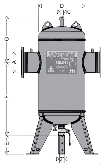
DN 200 - DN 300
